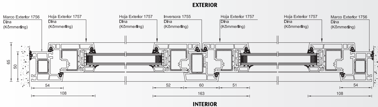
Corte B-B
