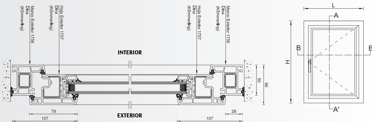
Corte A-A
