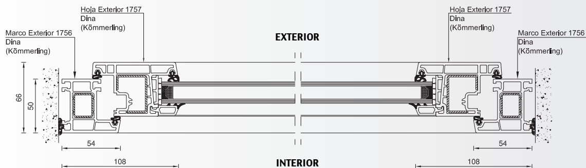
Corte B-B
